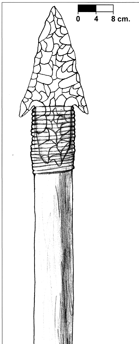
Fig. 5. Sistema de empuje propuesto para la punta de aletas y pedúnculo.
