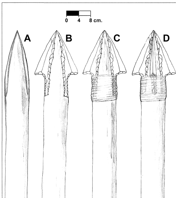
Fig. 6. Sistema de empuje propuesto para la punta de muesca. A: Cajeado del extremo distal del astil. B: Sujeción de los proyectiles en el astil mediante elementos adhesivos. C: Sujeción de los proyectiles en el astil mediante un amarre circular. D: Implementación de tres o cuatro elementos.
